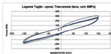
Fig. 2 - Prova per la determinazione del modulo G statico
