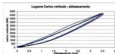
Fig. 1 - Prova per la determinazione della rigidità assiale
