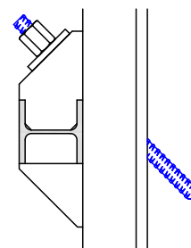
Geneigter Einbau inclined installation
