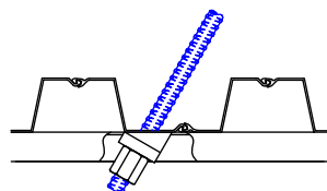
Schräger Einbau angular installation
